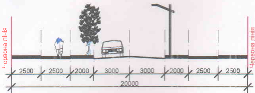
Поперчний профіль вул.Шевченка
