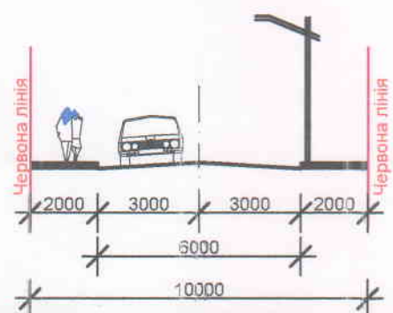
Поперчний профіль вул.Смерекової
